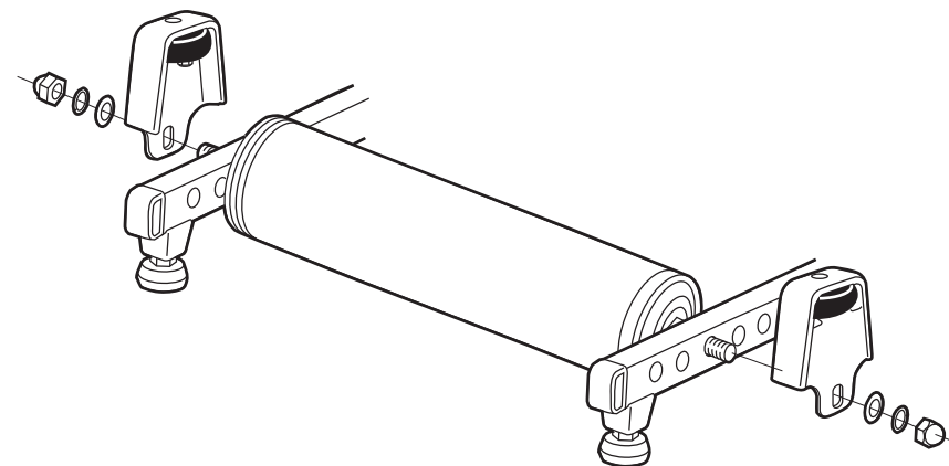
[組立図]
